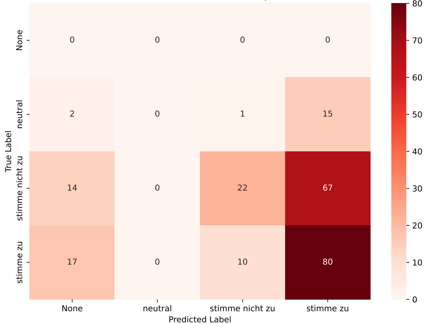
Confusion Matrix - Llama 2, temp: 0.3
